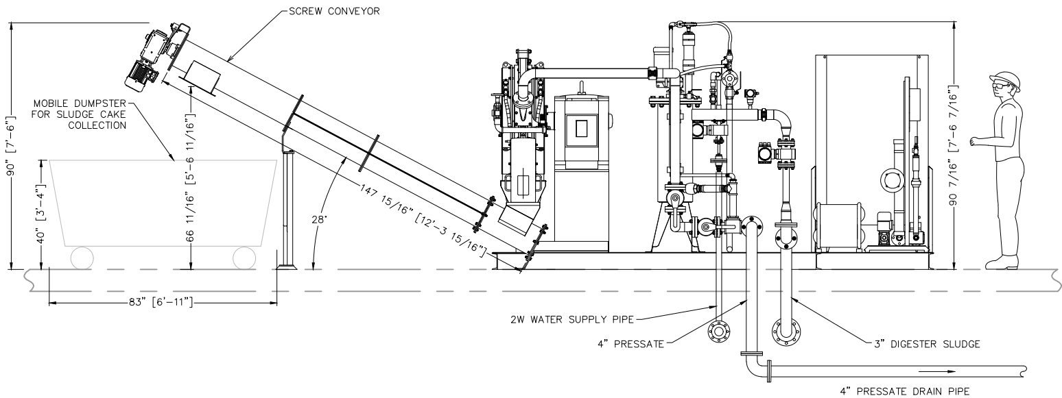
ROTARY FAN PRESS ELEVATION
